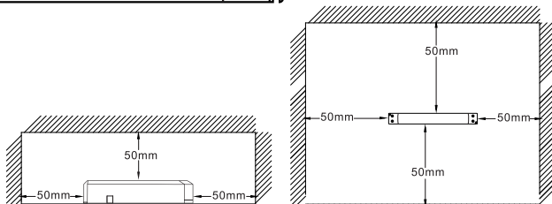
Sugerowany sposób montażu oraz przestrzeń wokół zasilacza
